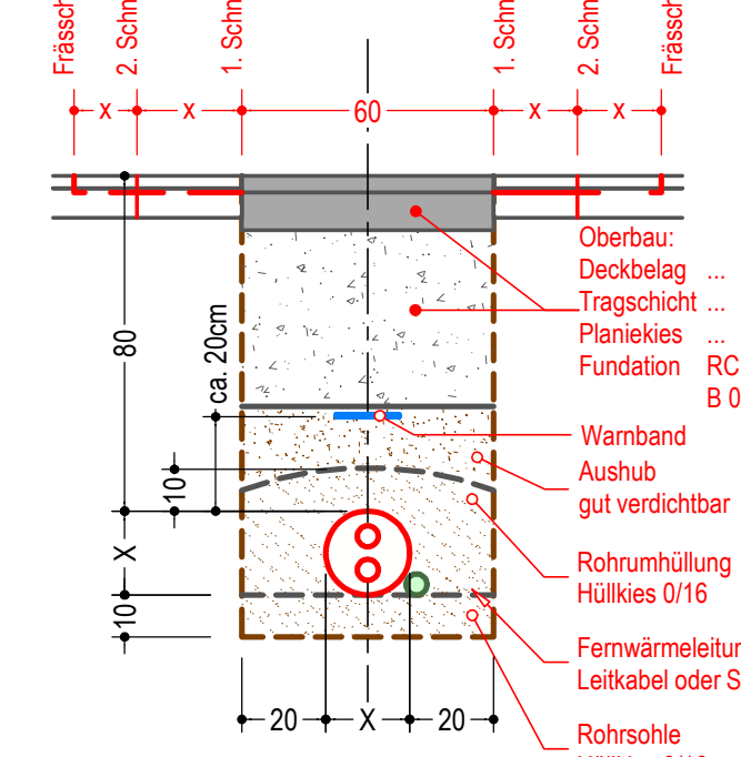
NP 2 1:20 DUO Vorplatz - Strassenbereiche
