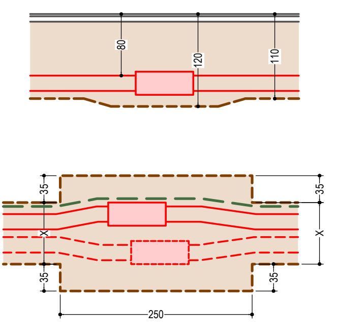
NP 2 1:20 DUO Vorplatz - Strassenbereiche
