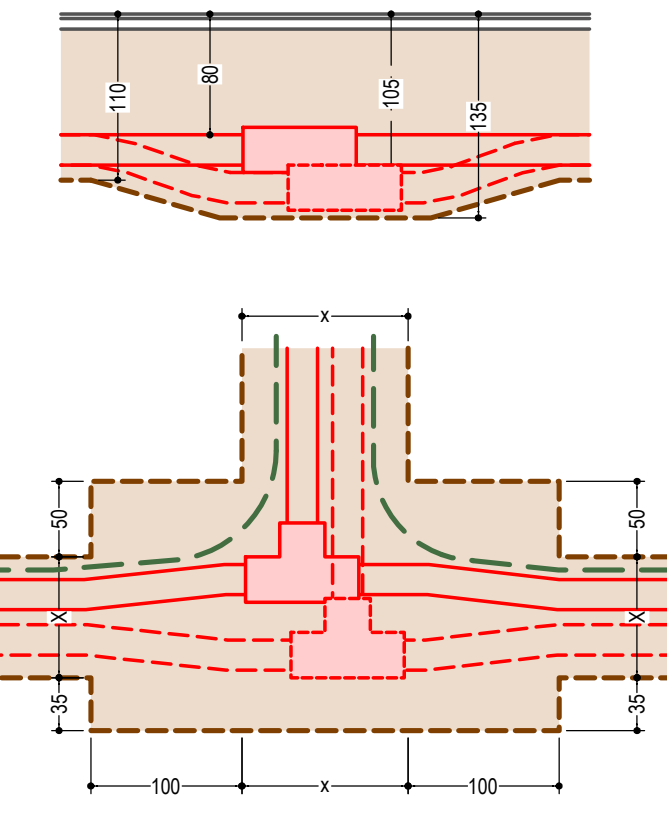
NP 1 1:20 DUO Feld - Wiesenbereiche
